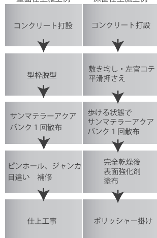
壁面仕上施工例
