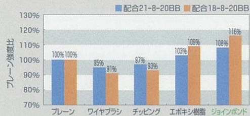
○各種工法によるせん断強度比 (20℃)
