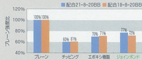
○各種工法による曲げ接着強度比 (20℃)
