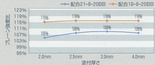
○ジョインボンド塗付厚さによるせん断強度比 (20℃)
