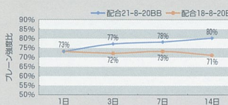
○打継コントロール時間別の曲げ接着強度比 (20℃)
